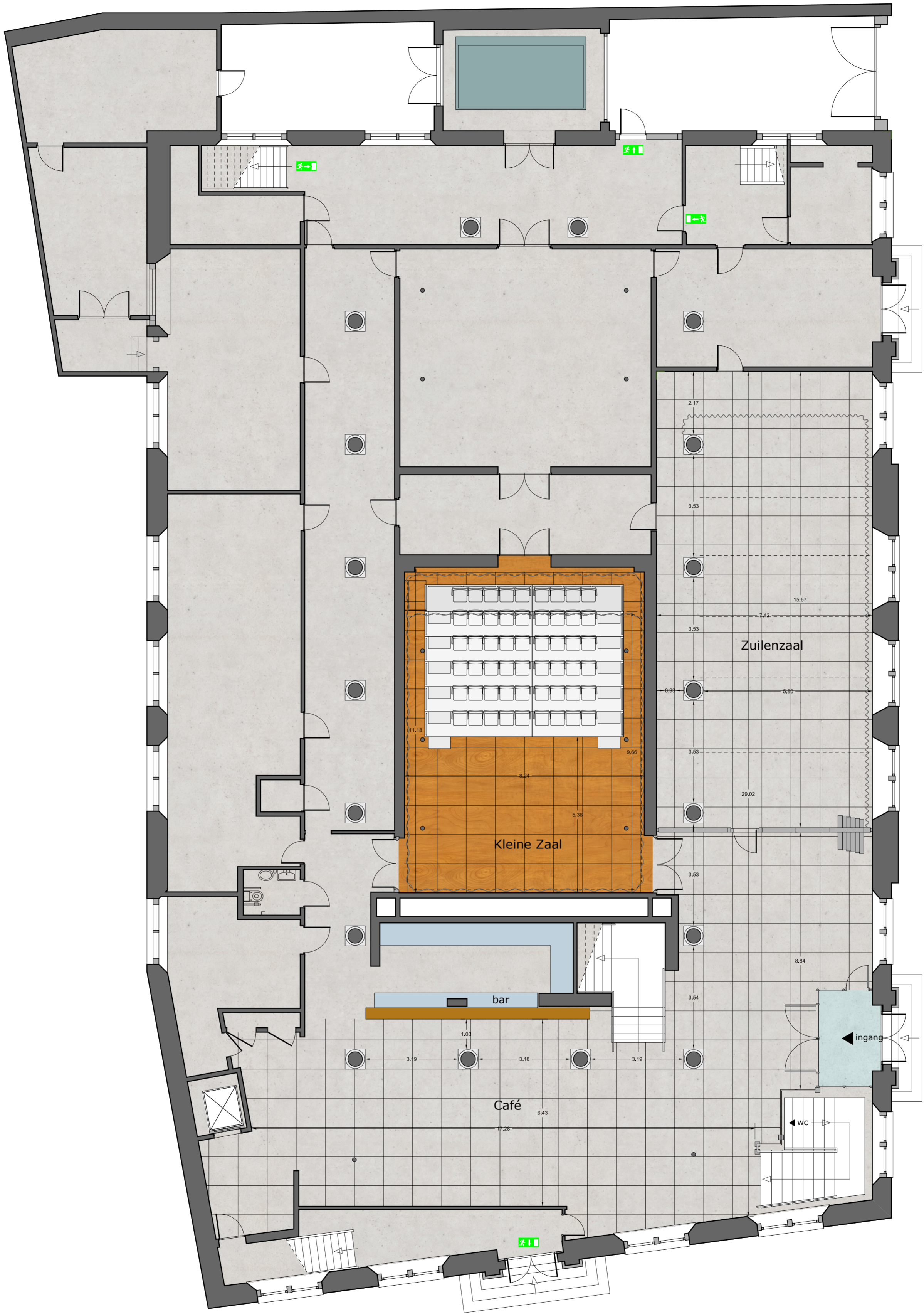
Compagnietheater begane grond schaal 1:100
