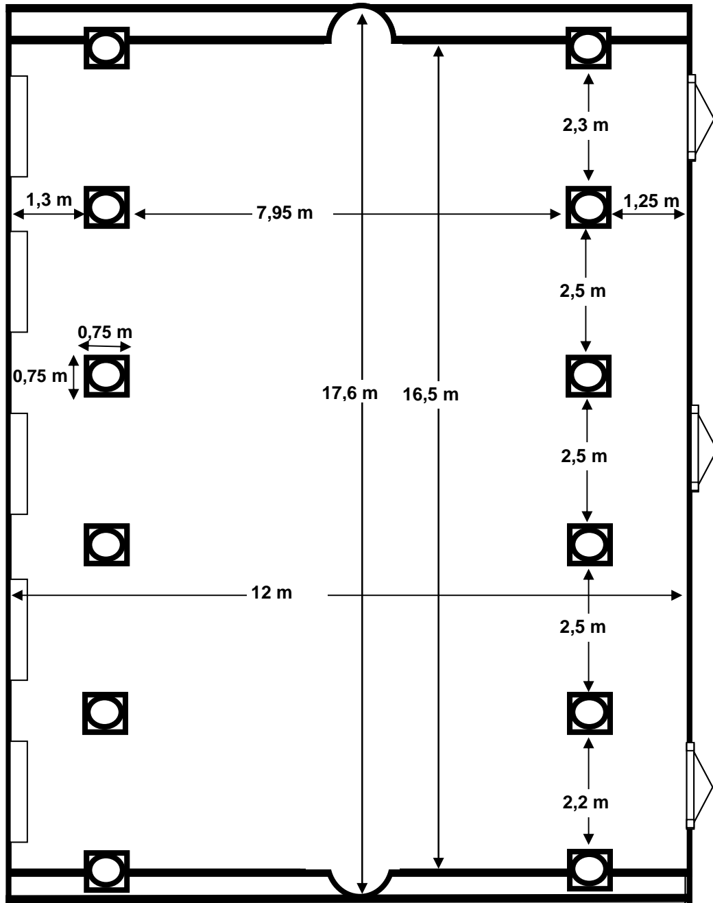
ZUILENZAAL MATEN SCHAAL 1-100
